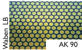
Waben LB 35 356 16 Dichroic (U 61-00) 1,5 mm BG: schwarz/black R: gold/gold
