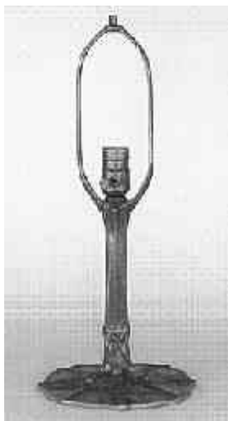
89 LB 461 PENGUIN FOOT BASE h: 43,0 cm / 17" für Schirmdurchmesser: 30 - 40 cm fits shades 12" - 16"
